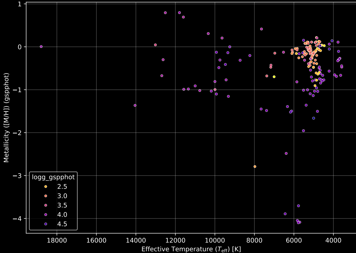
APOGEE DR17 Field: [203+04-RV_btx] Stellar Population Parameters (n= 185)
